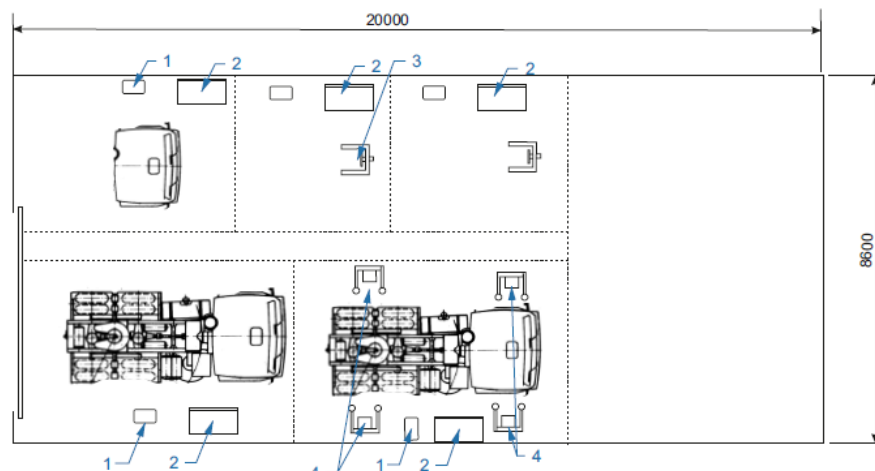
План застройки мастерской «Обслуживание грузовой техники»
